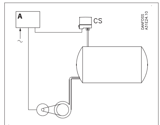
Beispiel 4 Steuerung einer Umwälzpumpe mit Druckschalter Typ CS über einen automatischen Stern-Dreieckschalter, Motorschuttschalter o.ä.
