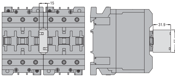
Verriegelungen G269 2
