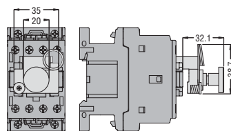
Manuelle Schließvorrichtung G454, G455
