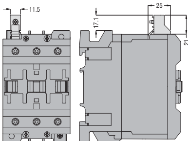
Hilfsklemmenblock G285
