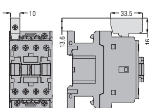
Klemmenblöcke G231 - 1 Pol
