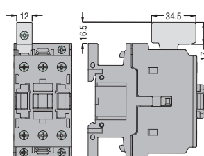
G232 - 1 Pol
