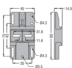
Schraubbefestigung BFX89 01
