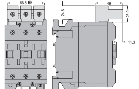
G271, G288 - 3 und 4 Pole
