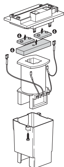
Spule komplett
