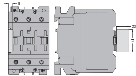
Entstörglieder G318, G319 225, G322
