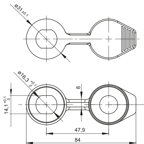
Pokrywa 2.904.008
