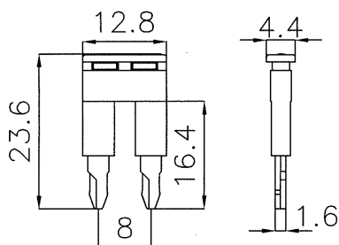
Zwieracz sprężynowy ZSN-6-2
