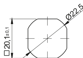
Otwór montażowy
